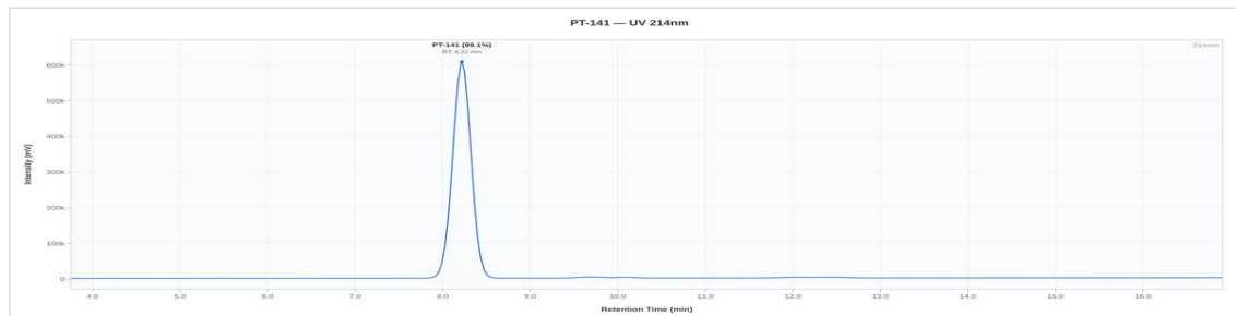
PT-141 10mg - 032026: UV Chromatogram
