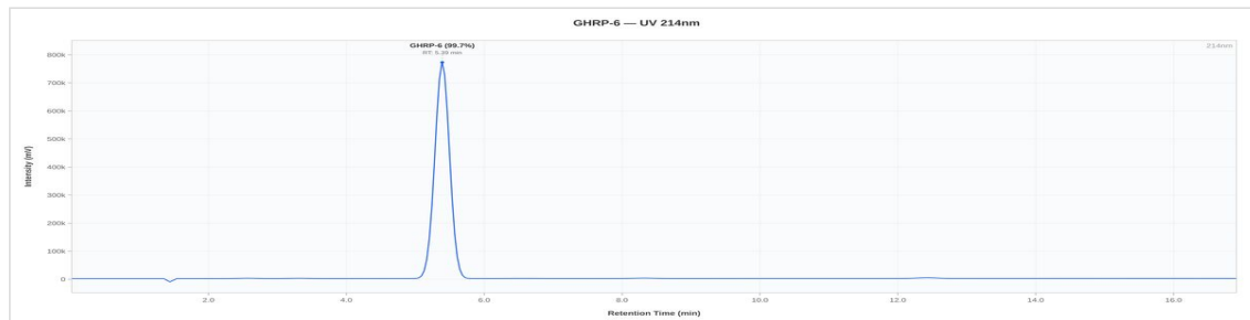
GHRP-6 10mg - 032026: UV Chromatogram
